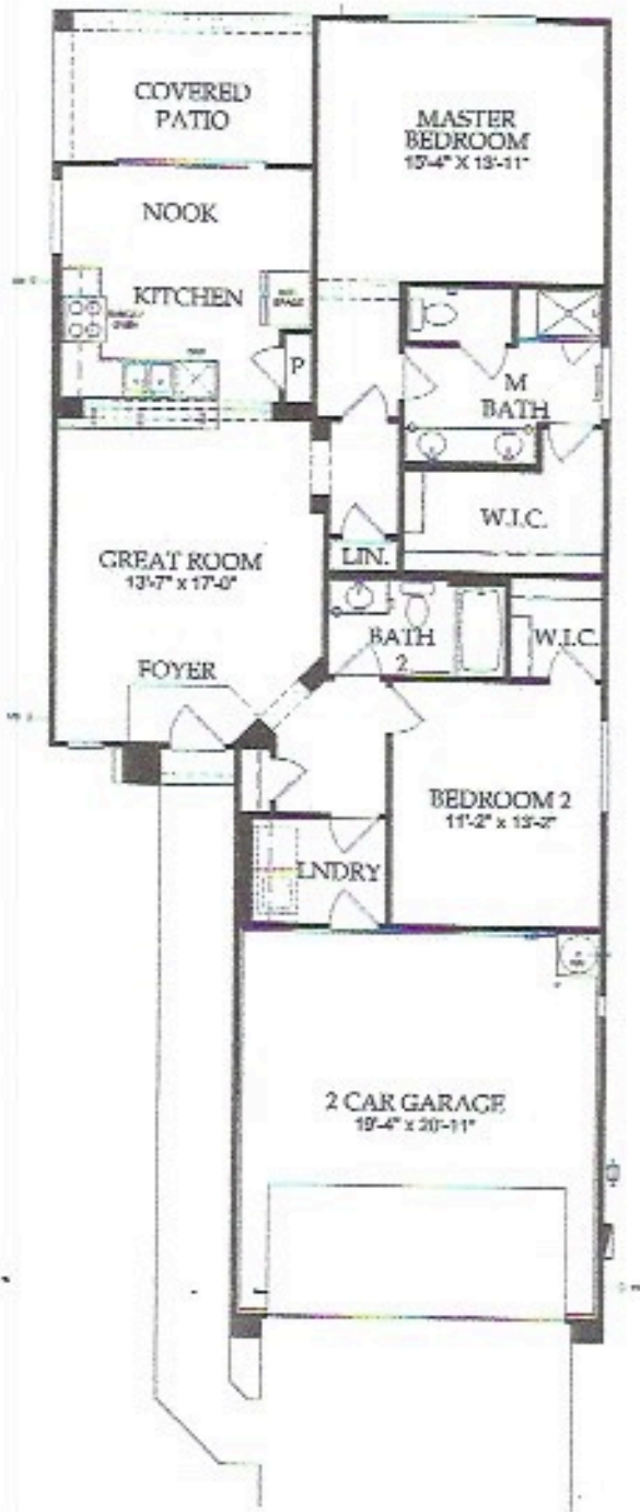
ELEVATION A
